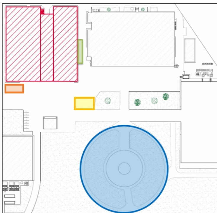
Planimetria dell'elissuperficie (evidenziata in blu), del fabbricato 24 (evidenziato in rosso), dell'area gestione carburanti (evidenziata in giallo), dell'area lavaggio elicotteri (evidenziata in arancione) e dell'area di stoccaggio serbatoi mobili (verde)
