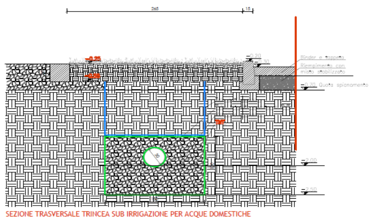
Figura 38: trincea drenante
